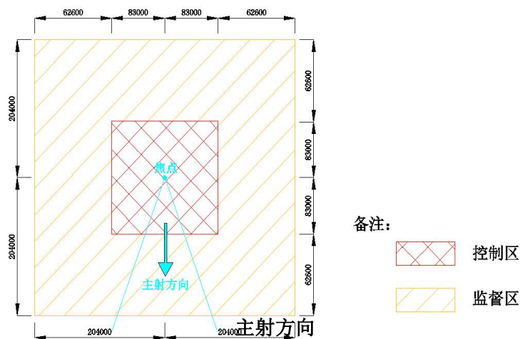
图 11-1 控制区、监督图划分示意图（XXG-3505 型定向 X 射线探伤机）
