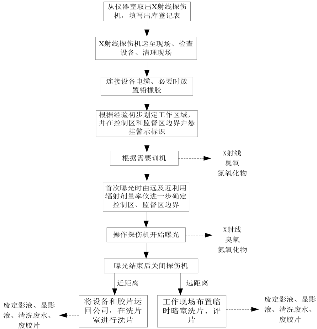
图 9-3 X 射线现场探伤工艺流程及产污环节示意图
